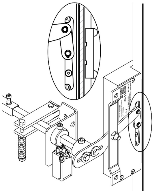
Abbildung 5: Position der Rollen
