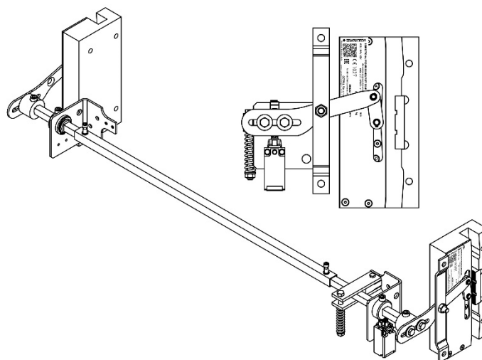
Abbildung 10: Synchronisation der Fangvorrichtungen mittels Auslösegestänge T-3
