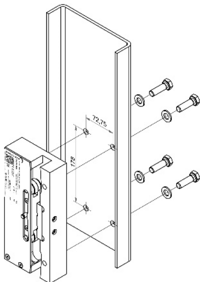
Abbildung 2: Einbau der Fangvorrichtung in den Rahmen (1)
