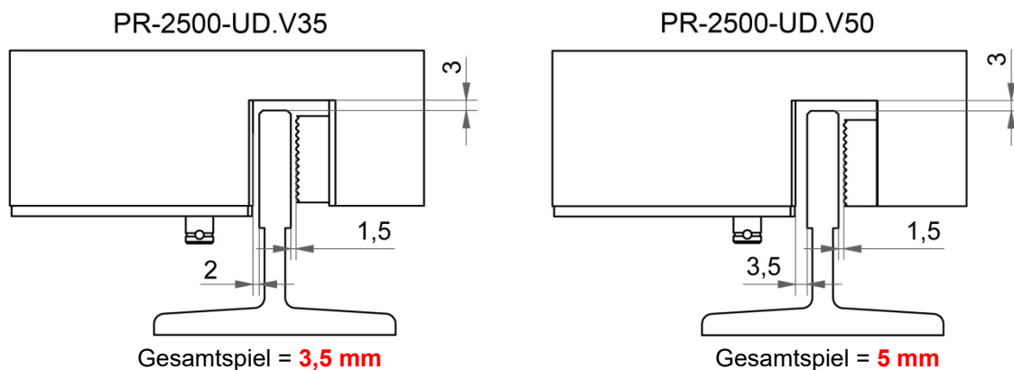
Abbildung 8: Justierung der Fangvorrichtung zur Führung
