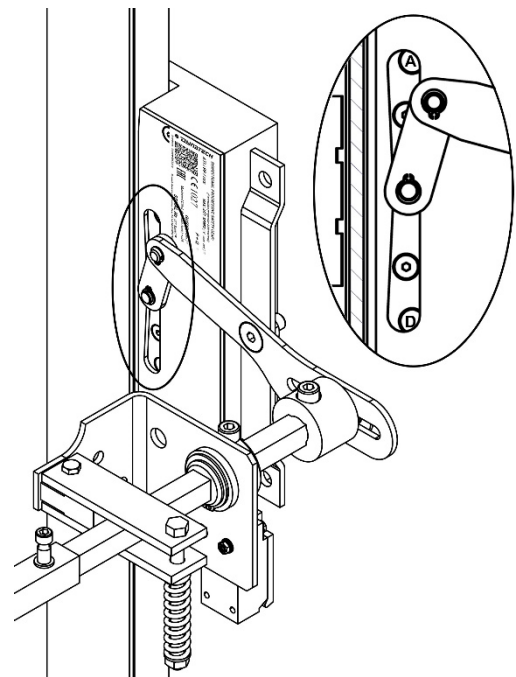
Abbildung 6: Position der Rollen an invertierten Führungen
