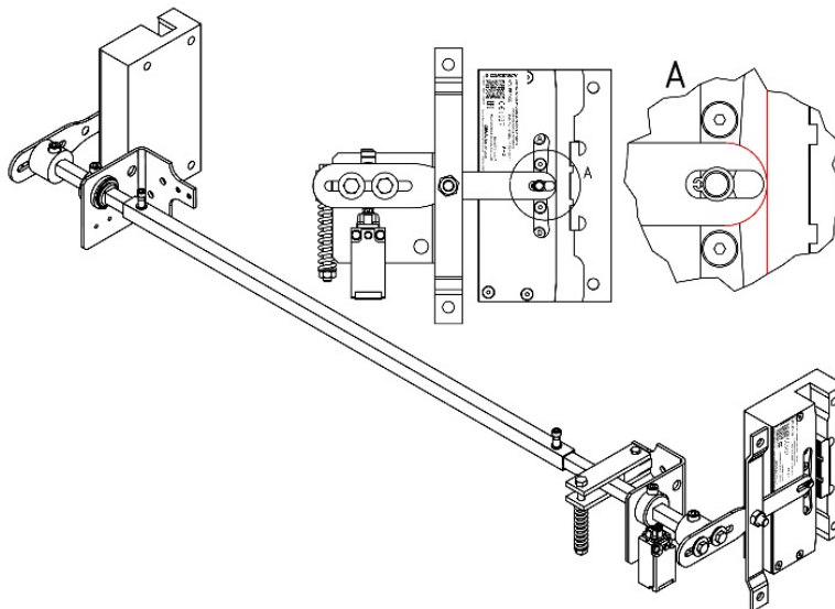
Abbildung 9: Synchronisation der Fangvorrichtungen mittels Auslösegestänge T-2
