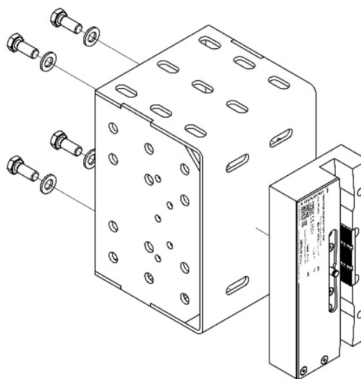
Abbildung 3: Einbau der Fangvorrichtung in den Rahmen (2)
