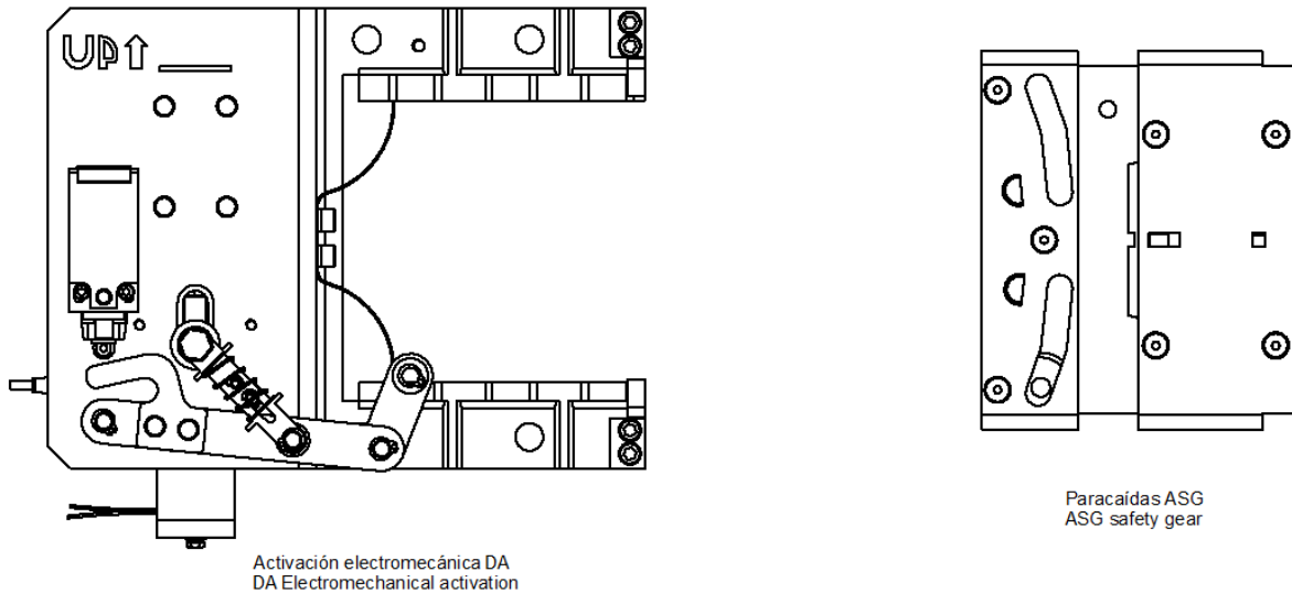
Imagen 2. Diferenciación entre activación y paracaídas
