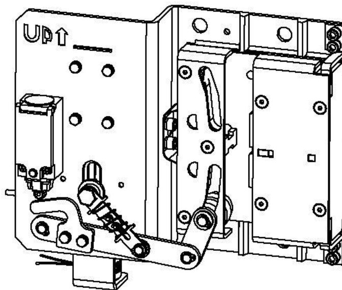
Imagen 1 Paracaídas electromecánico unidireccional eASG
